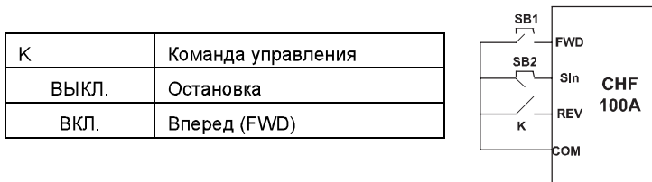
Рисунок 6.13. Трехпроводное управление режим 1.
