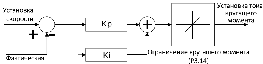
Рисунок 6.6. Схема регулятора скорости ASR
