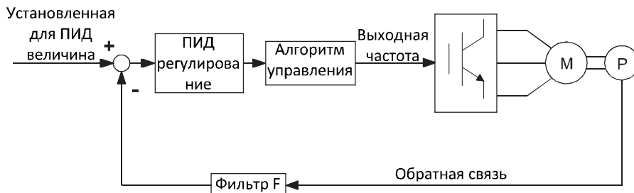
Рисунок 6.24. Блок-схема ПИД регулирования.
