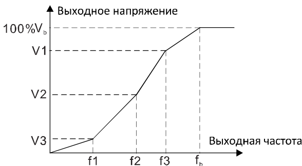
Рисунок 6.10. Установка параметров для пользовательской вольт-частотной характеристики
