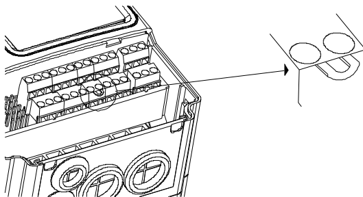
Рисунок 4.13. U-образная перемычка.
