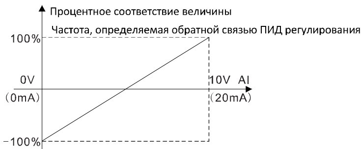
Рисунок 6.15. Отношение между сигналом аналогового входа AI и соответствующей величиной.
