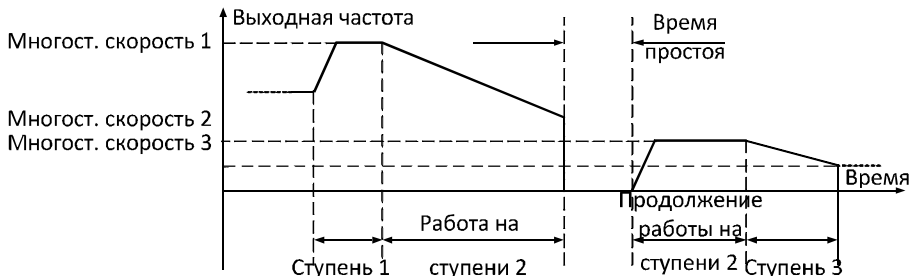
Рисунок 6.31. Кривые защиты двигателя от перегрузки по току.
