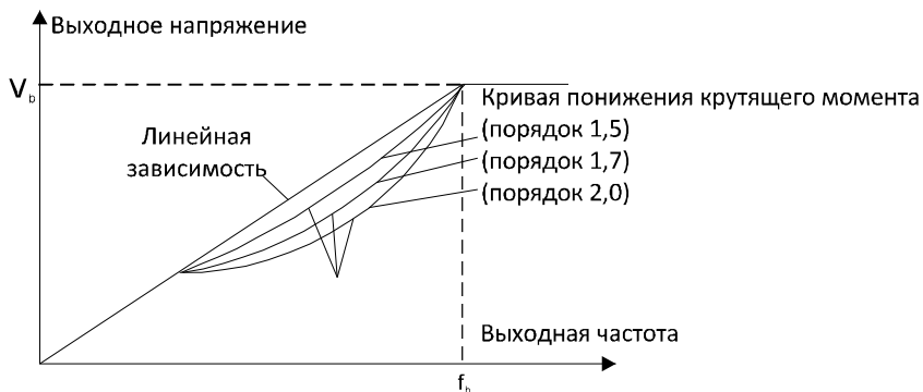
Рисунок 6.8. Вольт-частотная характеристика
