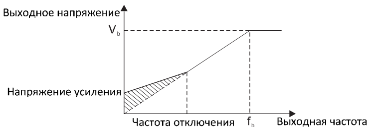
Рисунок 6.9. Характеристика для «ручного» усиления крутящего момента
