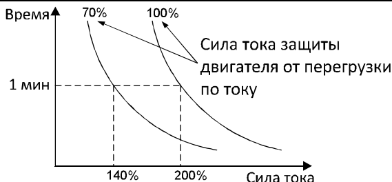
Рисунок 6.32. Кривые защиты двигателя от перегрузки по току.
