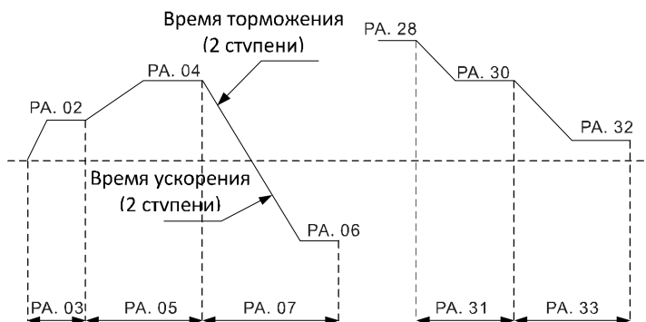
Рисунок 6.29. График работы с простым ПЛК.
