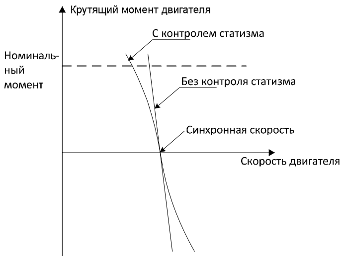
Рисунок 6.23. Контроль статизма.
