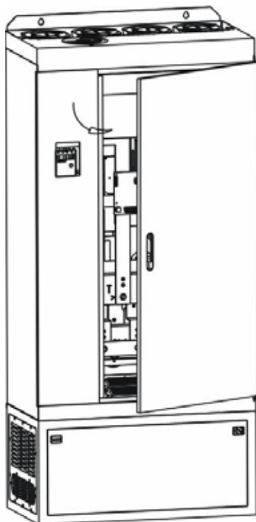
Рисунок А. 15. Открытие шкафа инвертора
