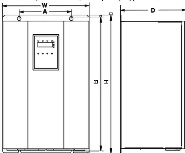
Рисунок А. 2. Габаритные размеры (18.5–110 кВт)
