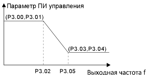
Рисунок 6.7. Диаграмма параметров ПИ управления
