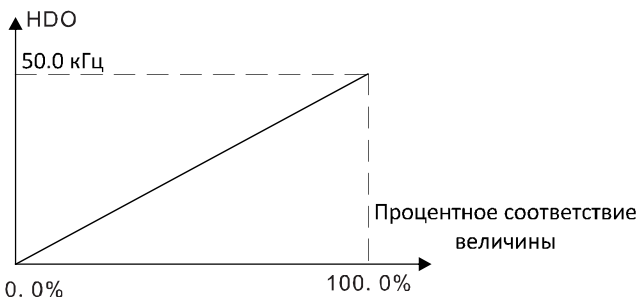
Рисунок 6.17. Отношение между сигналом выхода HDO и соответствующей величиной.
