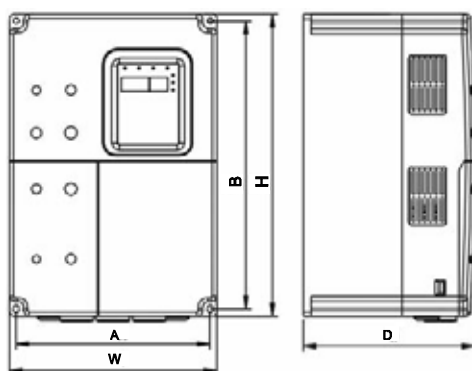
Рисунок А. 4. Габаритные размеры (до 7.5 кВт включительно)
