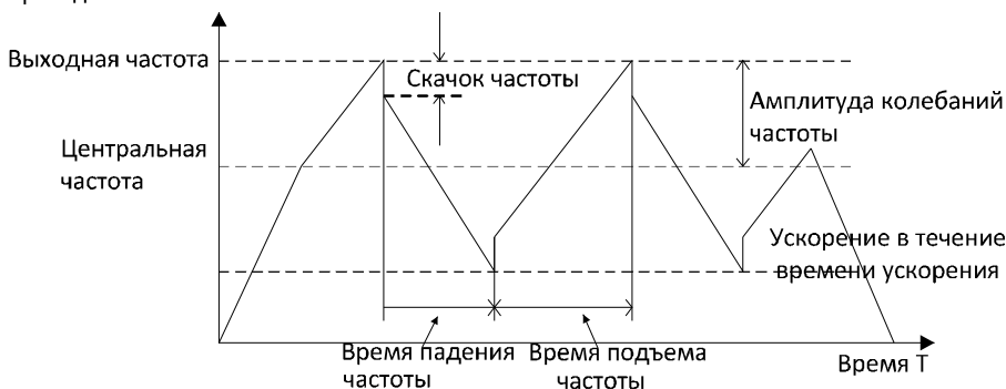
Рисунок 6.19. График управления двигателем с колебаниями частоты.
