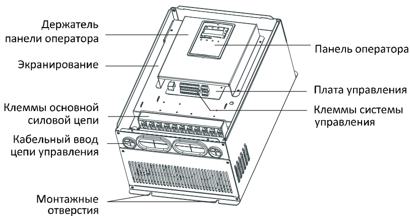
Рисунок 1.2. Компоненты инверторов (15 кВт и меньше)
