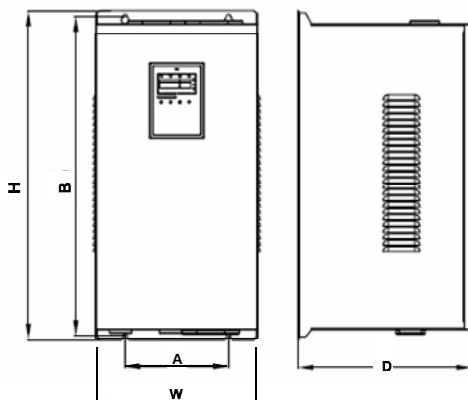
Рисунок А. 6. Габаритные размеры (22–55 кВт)
