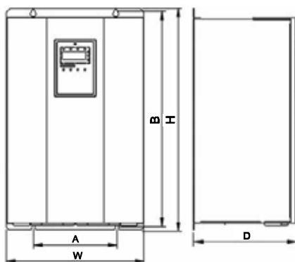
Рисунок А. 5. Габаритные размеры (11–18.5 кВт)
