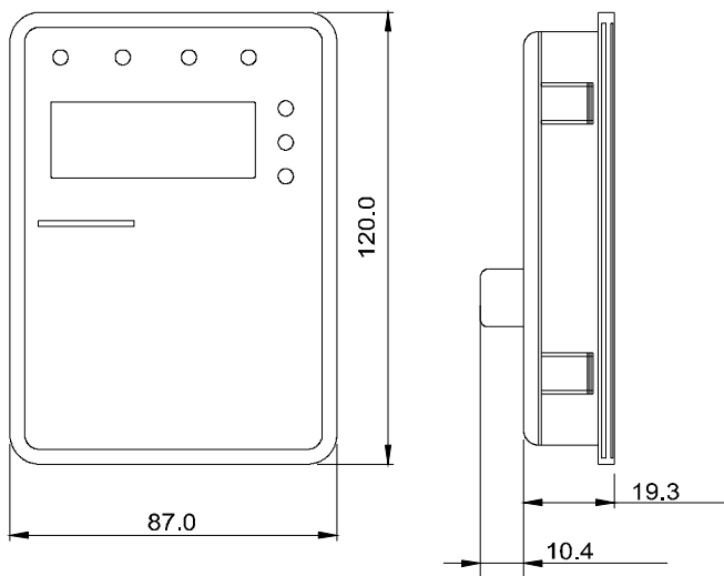
Рисунок А. 11. Габаритные размеры большой панели
