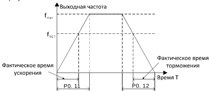
Рисунок 6.1. Времена ускорения/торможения
