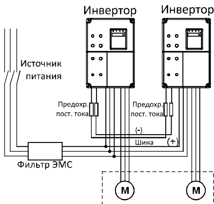
Рисунок 4.19. Электромонтаж общей шины постоянного тока
