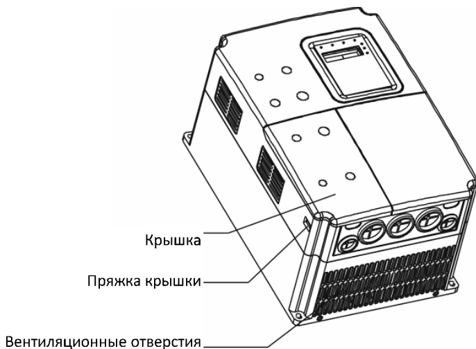
Рисунок 1.2. Компоненты инверторов (15 кВт и меньше)
