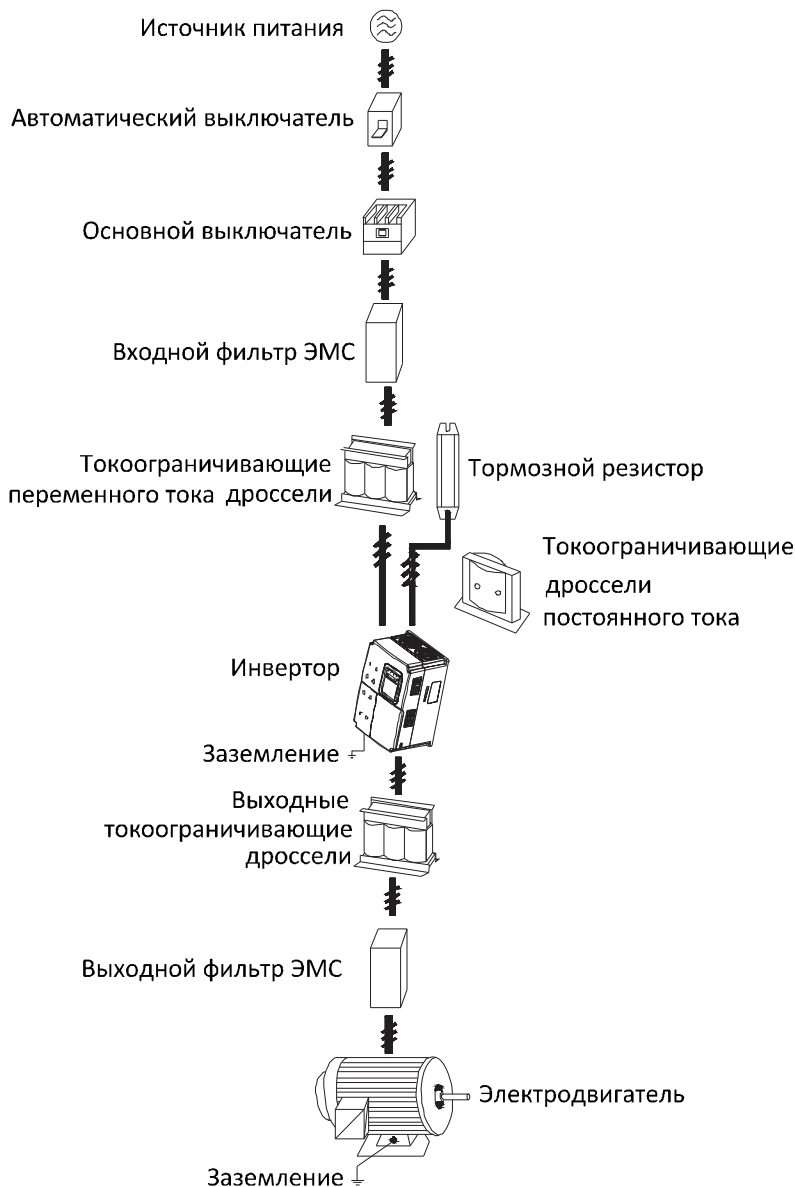
Рис. 4.1. Подключение периферийных устройств
