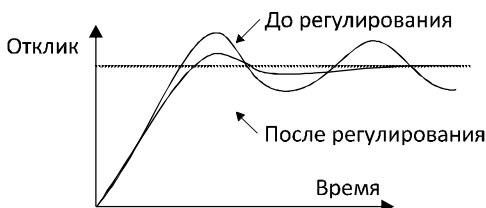
Рисунок 6.26. Подавление низкочастотных осцилляций.
