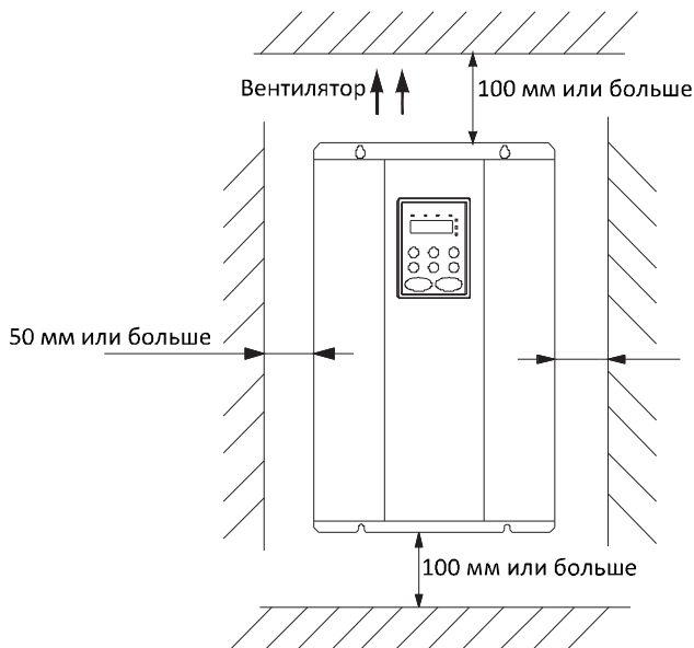
Рисунок А. 8. Безопасные дистанции до предметов
