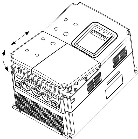
Рисунок А. 13. Снятие пластиковой крышки
