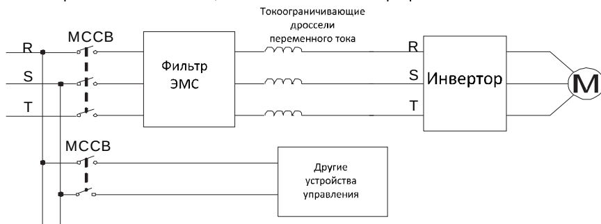
Рисунок 4.16. Электромонтаж входной силовой цепи
