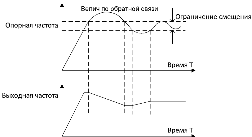
Рисунок 6.28. Отношения ограничения смещения и выходной частоты.
