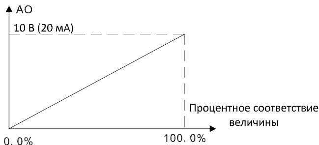
Рисунок 6.16. Отношение между сигналом выхода АО и соответствующей величиной.
