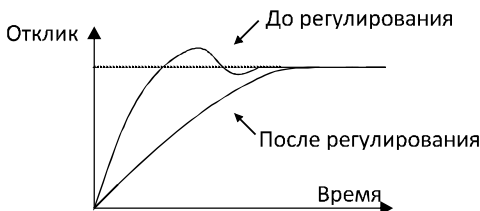
Рисунок 6.25. Подавление переуправления.
