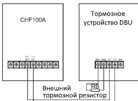
Рисунок В. 2 Подсоединение тормозного устройства
