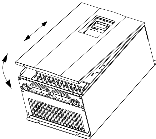
Рисунок А. 14. Снятие металлической крышки
