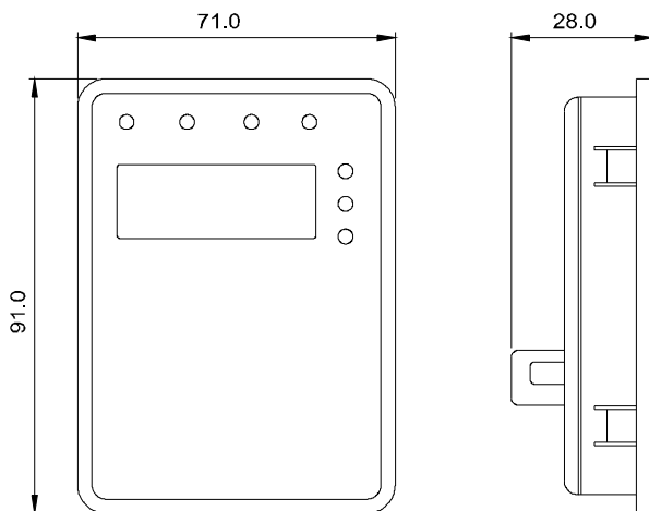
Рисунок А. 9. Габаритные размеры малой панели
