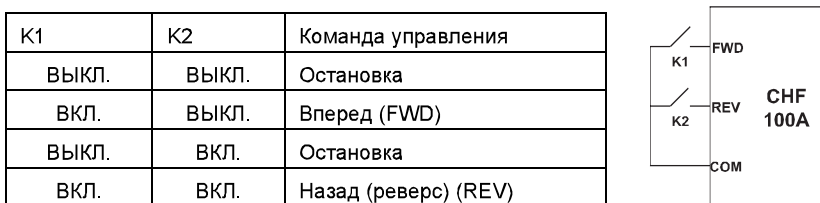
Рисунок 6.12. Двухпроводное управление режим 2.
