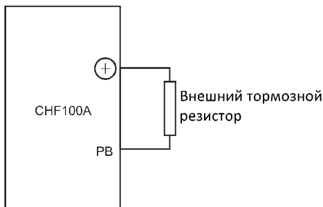
Рисунок В. 1 Подсоединение тормозного резистора
