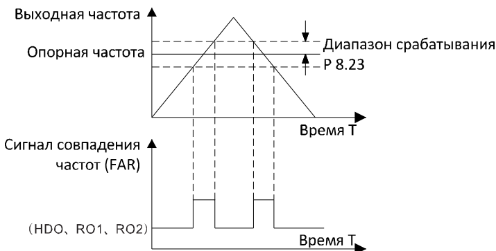
Рисунок 6.22. График сигнала совпадения частот (FAR).
