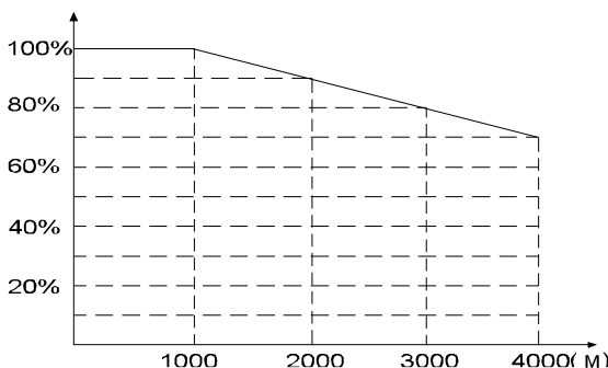
Рисунок 3.1. Соотношение между выходной силой тока и высотой установки
