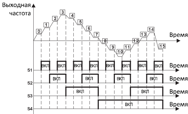
Рисунок 6.30. Схема многоступенчатого регулирования скорости.
