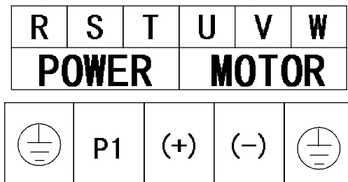
Рисунок 4.5. Клеммы силовой цепи (132–315 кВт)
