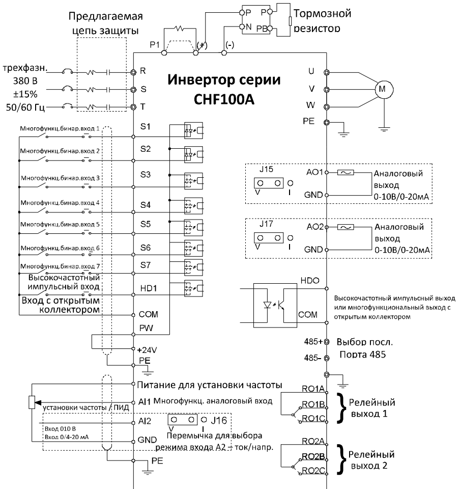
Рисунок 4.12. Типовая схема подключения
