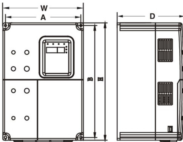
Рисунок А. 1. Габаритные размеры (до 15 кВт)
