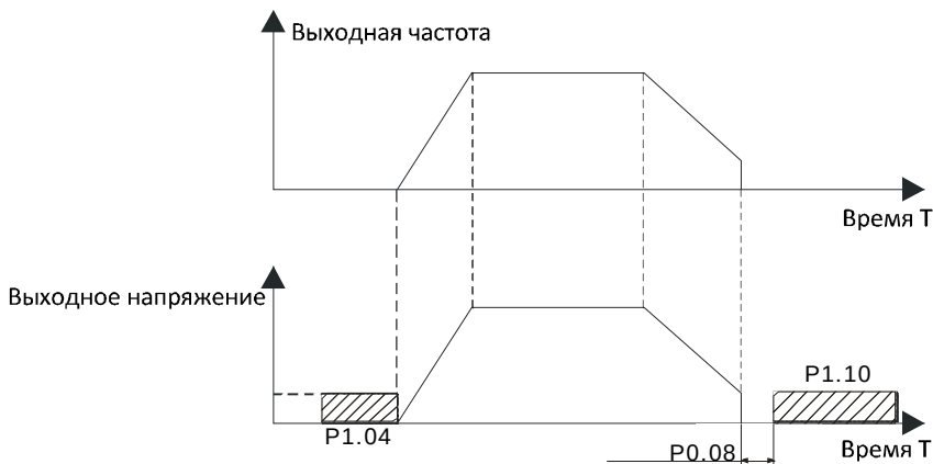
Рисунок 6.4. Диаграмма торможения постоянным током
