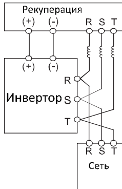
Рисунок 4.18. Электромонтаж цепи рекуперации
