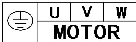
Рисунок 4.10. Клеммы силовой цепи (22 кВт и выше)
