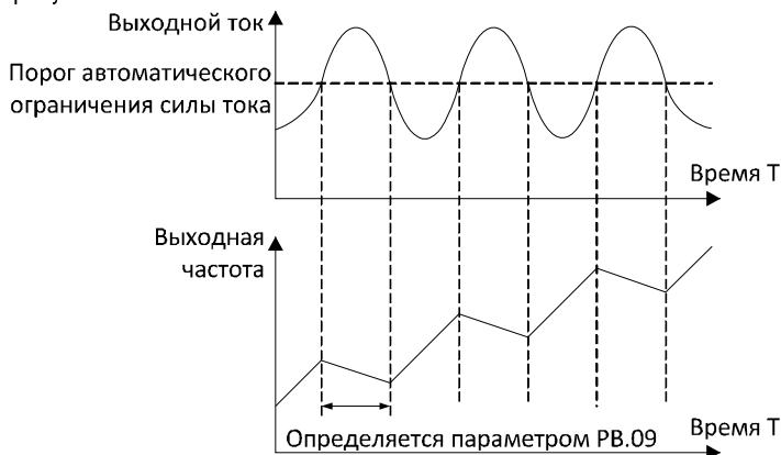
Рисунок 6.34. Функция защиты от сверхтоков.
