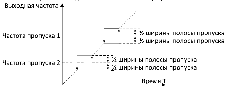
Рисунок 6.18. График пропуска частот.
