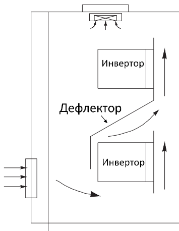
Рисунок А. 7. Установка нескольких инверторов
