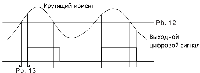
Рисунок 6.35. Функция ограничения крутящего момента.
