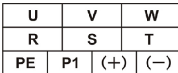
Рисунок 4.6. Клеммы силовой цепи (350–630 кВт)
