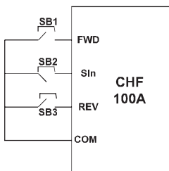
Рисунок 6.14. Трехпроводное управление режим 2.
