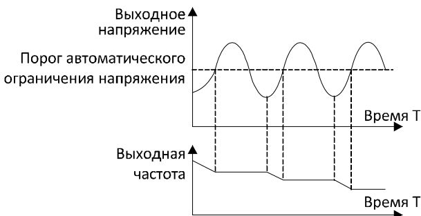
Рисунок 6.33. Функция защиты от перенапряжения.
