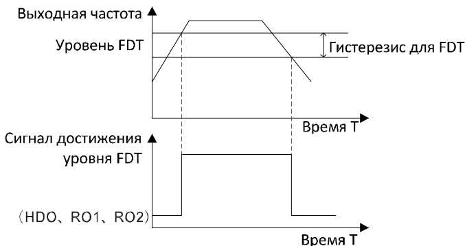
Рисунок 6.21. Уровень FDT и гистерезис FDT.
