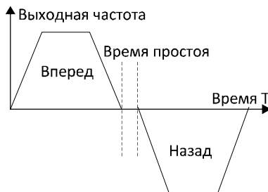
Рисунок 6.5. График задержки переключения вперед-назад (FWD/REV)
