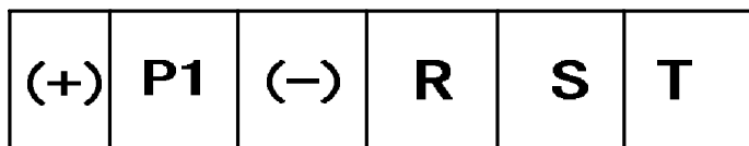
Рисунок 4.9. Клеммы силовой цепи (11–18.5 кВт)
